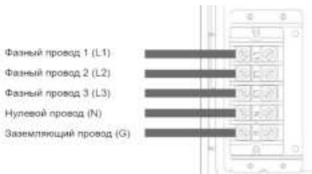
Рис.9. Подключение прибора
