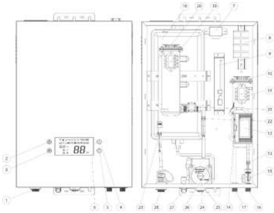
Рис. 1. Конструкция изделия
