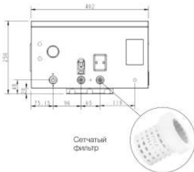
Рис. 13. Сетчатый фильтр
